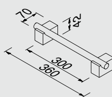
917506-02 Badgreep 30 cm Grab rail 30 cm Wannengriff 30 cm Poignée de bain 30 cm Поручень 30 см
