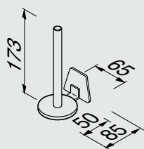
915126 Reserverolhouder, dubbel Spare roll holder, double Reserverollenhalter, doppelt Porte-papier rouleau de réserve, double Держатель запасного рулона двойной
