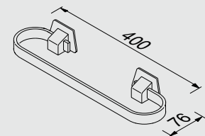
915121-40 Wandhanddoekhouder 40 cm Towel rail 40 cm Wandhandtuchhalter 40 cm Porte serviettes 40 cm Настенный полотенцедержатель 40 см
