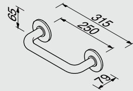
91131-25 Badgreep 25 cm 20 mm buis, verdeckte bevestiging Grab rail 25 cm 20 mm tube, concealed fixing Wannengriff 25 cm, 20 mm Rohr, verdeckte Befestigung Poignée de bain 25 cm, 20 mm tube, fixation couverte Поручень 25 см, диаметр трубки 20 мм, скрытое крепление
