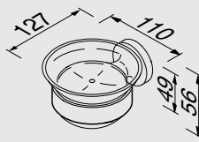
917303-02 Zeephouder Soap holder Seifenhalter Porte-savon Мыльница
